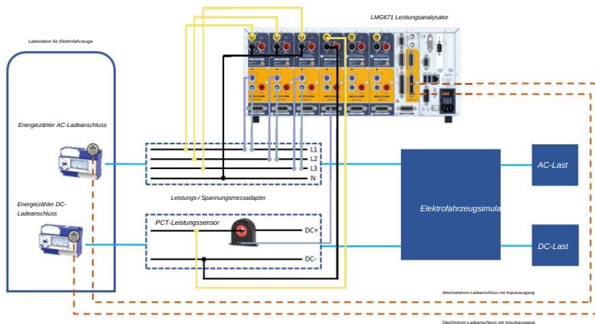
Messaufbau mit LMG671 und PCT-Stromsensor
