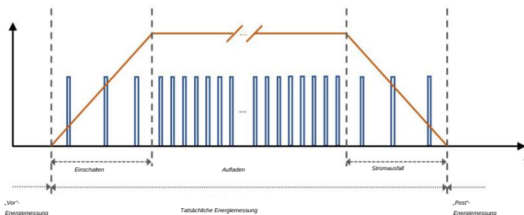
Vom Leistungsanalysator LMG600 erfasste Energiezählerimpulse und gemessene Energie
