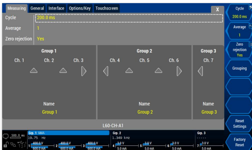
LMG600 mit 7 Leistungskanälen, organisiert in 3 Gruppen
