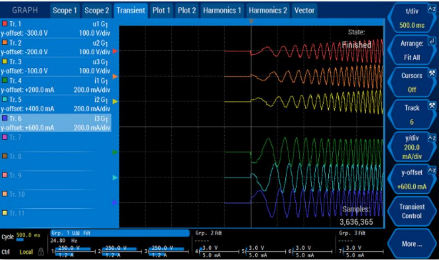
Screenshot der Event-Trigger-Option mit bis zu 16 Millionen Samples. Die Scope View bietet eine schnelle und komfortable Möglichkeit, Signale im Zeitbereich zu visualisieren. Mit dem Viewer für den Event-Trigger können Sie das Verhalten von Spannung, Strom, Leistung oder anderen Variablen in 16 Spuren aus verschiedenen Kanälen grafisch und mit variabler Zeitbasis anzeigen. Mit Cursors können Segmente markiert oder Zeit- und Amplitudenunterschiede zwischen zwei Punkten gemessen werden. Der Kehrwert der Zeitdifferenz (also die Frequenz) wird ebenfalls angegeben. Eine weitere Analyse der Proben kann am PC mit der LMG Sample Vision-Software durchgeföhrt werden.
