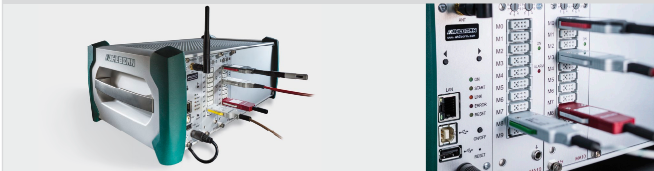
Anschlüsse für ALMEMO® Fühler und für Vernetzung (OLED Statusanzeige)
