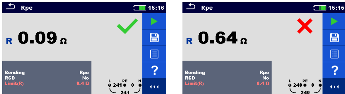
Abbildung 7.76: Beispiele für Ergebnisse der Schutzleiterwiderstandsmessung
