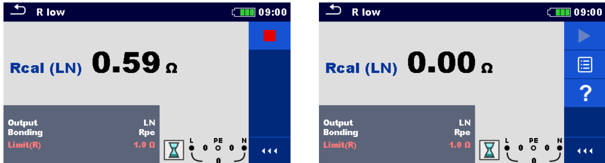
Abbildung 7.21: Ergebnisse mit alten und neuen Kalibrierungswerten
