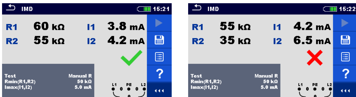
Abbildung 7.73: Beispiele für Ergebnisse der IMD Prüfung
