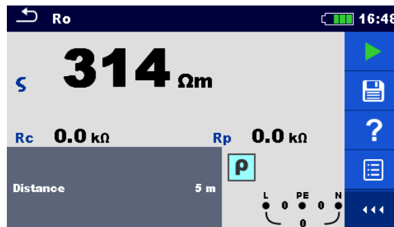
Abbildung 7.57: Beispiele für Ergebnisse der Messung des spezifischen Erdwiderstands
