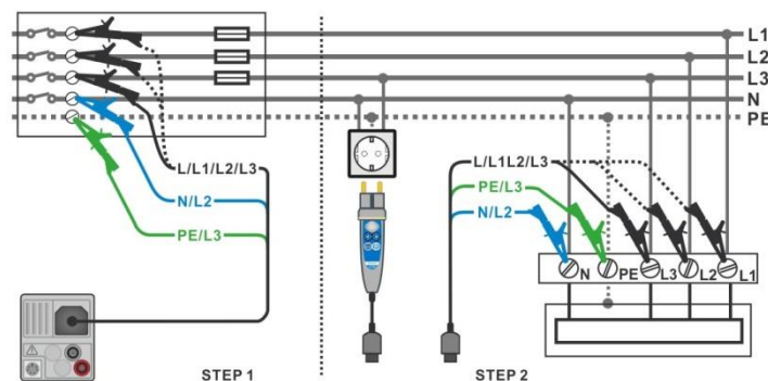
Abbildung 8.4: AUTO TT Messung
