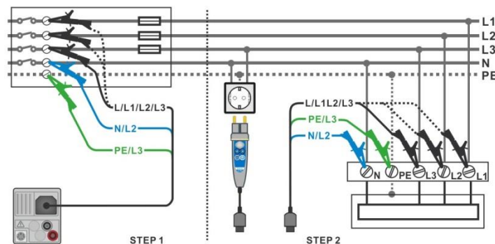
Abbildung 7.45: Spannungsabfallmessung – Anschluss des Commander-Prüfstecker und der Dreileiter-Prüfleitung
